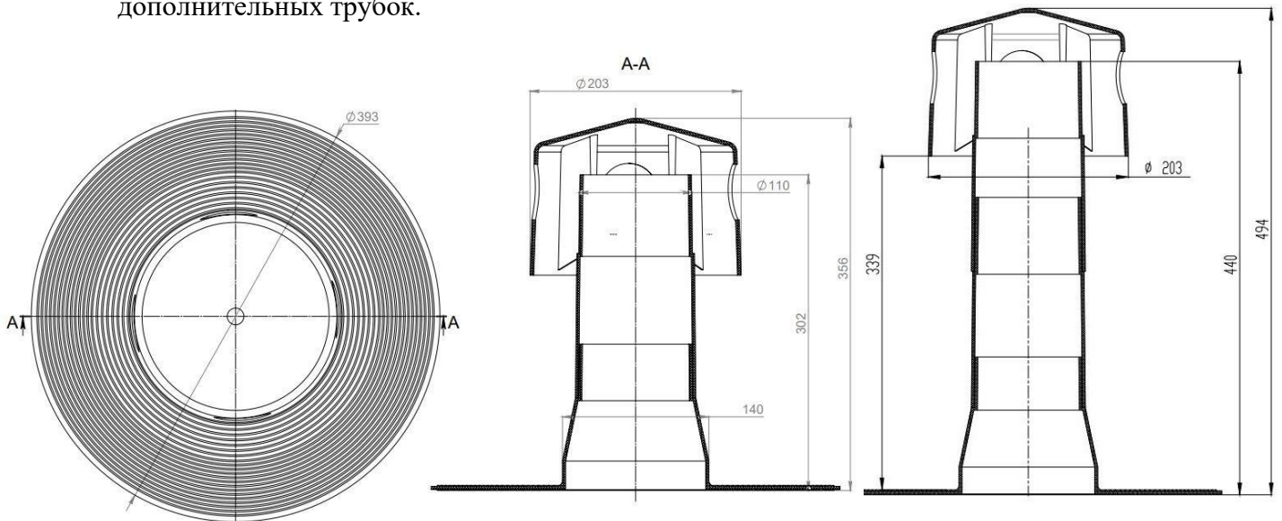
Рис. 1. Схема аэратора
